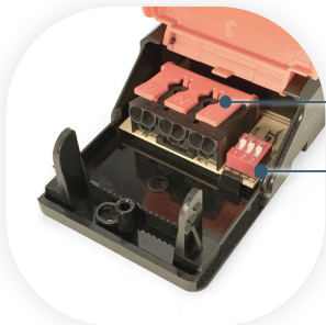
ANSCHLUSSRAUM
